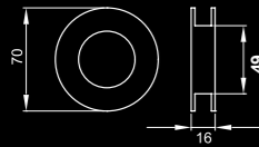
Schiebetürmuschel für Glastür EZ1706 GS – EZ1706 GSH (verschraubbar) Bohrdurchmesser im Glas: 50 mm, TS: 8-11 mm Farbe: Edelstahl matt
