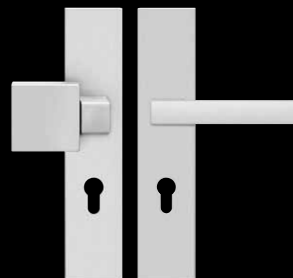
Edelstahl Schutzbeschlag rechteckig – ESG 675 Q Schutzklasse 2 nach DIN EN 1906 und Einbruchsicherheit 1 nach DIN 18257
