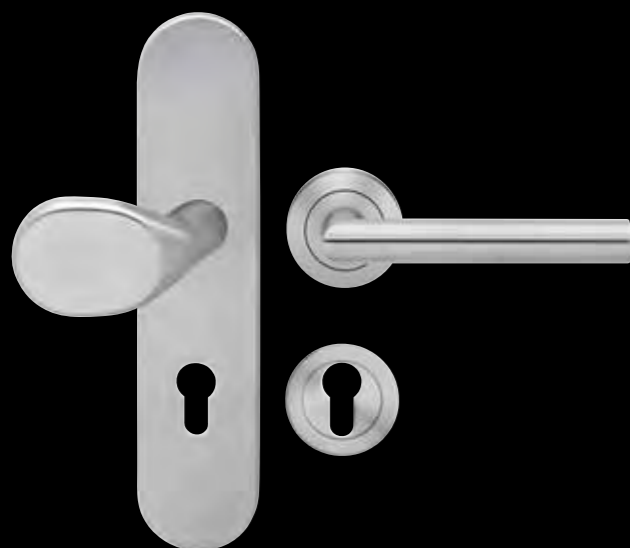
Edelstahl Kombi-Schutzbeschlag ESGR 670 K (kleine Abb) Einbruchsicherheit Klasse 0 Ausführung wie oben mit Kernziehschutz Zylinderüberstand 10 – 15 mm ab Türblatt Farbe: Edelstahl matt
