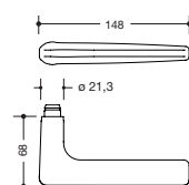
Modell 261X
