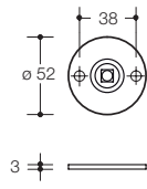
Drückerrosette 305.21XAL
