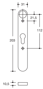
Schild 217...
