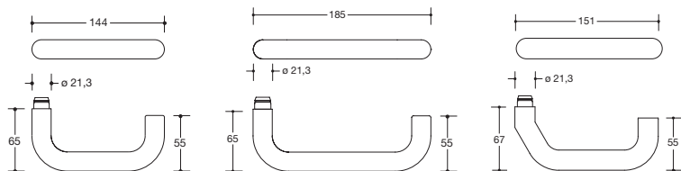
Modell 111X
