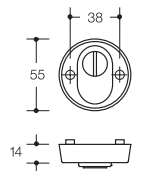
Schutzrosette 306.23X..ESZ..
