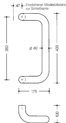
HEWI Griff ø 40 mm · aus hochwertigem Polyamid, Achsmaß 360 mm
