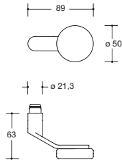
Modell 106X
