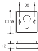
Schutzrosette 308X..ES..
