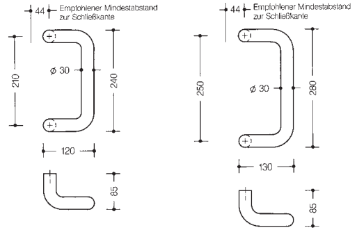
HEWI Griff ø 30 mm · aus hochwertigem Polyamid
