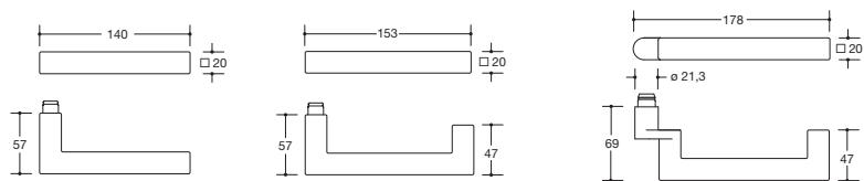
Modell 101X
