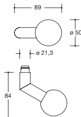
Modell 108X
