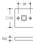
Drückerrosette 307...SX..
