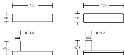
Modell 185X
