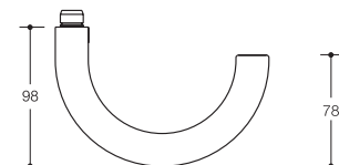
Modell 115.23
