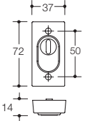
Schutzrosette 318X..ESZ
