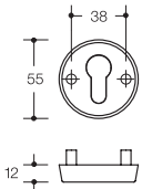
Schutzrosette 306.23X..ES..
