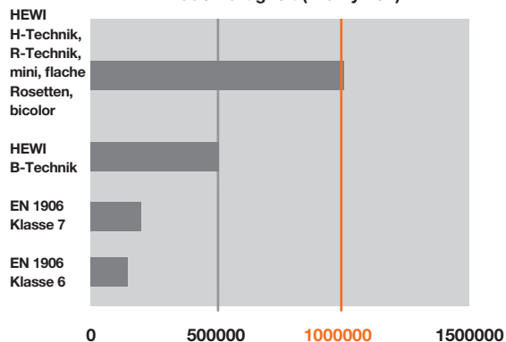
Dauerhaftigkeit (Prüfzyklen)
