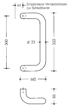
HEWI Griff ø 33 mm · aus hochwertigem Polyamid, Achsmaß 300 mm
