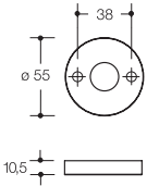
Drückerrosette 305...X..
