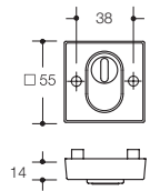
Schutzrosette 308X..ESZ..
