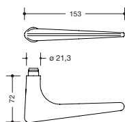
Modell 251X
