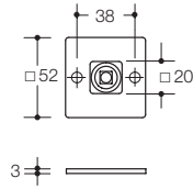
Drückerrosette 307.20SXAL
