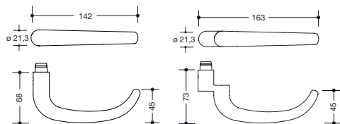
Modell 173X
